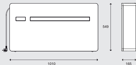
SC21DCIN, SC23DCIN(1000)
